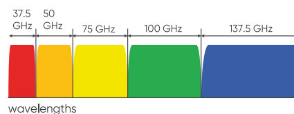
Рисунок 1 – Фиксированная (Fixed Grid) и гибкая (Flex Grid) частотные каналные сетки
