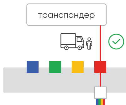
Рисунок 2 – Изменение длины волны канала на транспондере для «Colored» и «Colorless» систем ROADМ:
