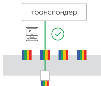
Рисунок 2 – Изменение длины волны канала на транспондере для «Colored» и «Colorless» систем ROADМ:
