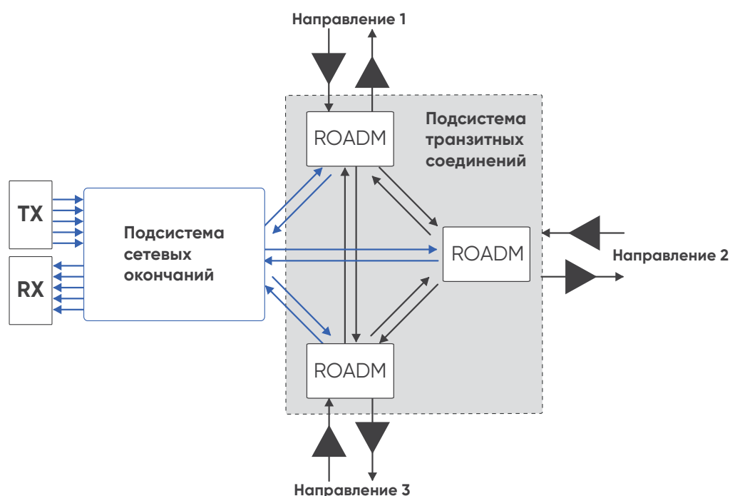
Рисунок 5 – Функциональная схема трехсвязного транзитно-оконечного узла ввода/вывода ROADM с подсистемами транзитных соединений и сетевых окончаний
